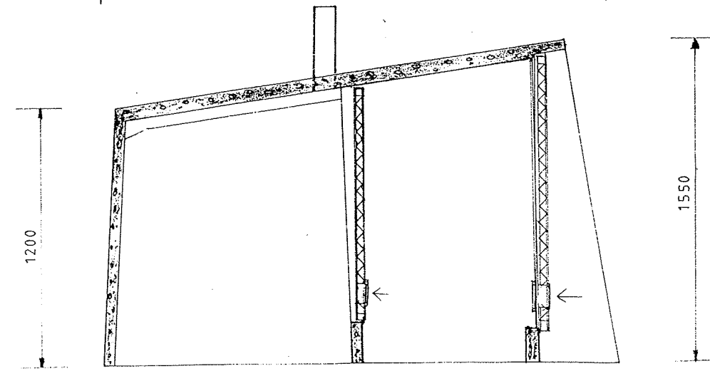
C-C
